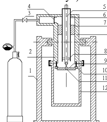
Рисунок 3 – Схема експериментальної установки
