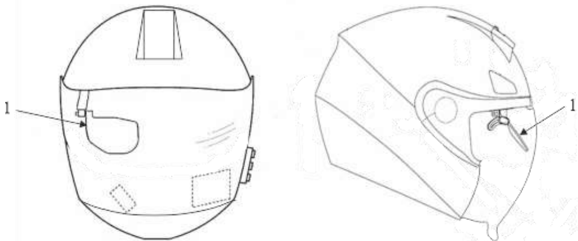
Рисунок 1 – Розміщення проєкційного дисплею на захисному шоломі військовослужбовця (1 – проєкційний дисплей)
