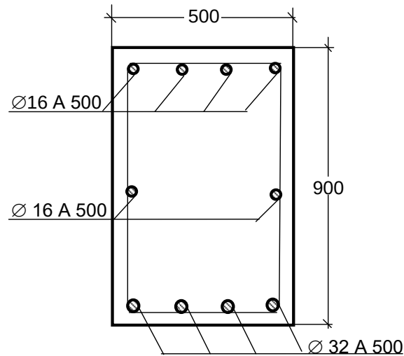
Рисунок – 1 Параметри перерізу та схема армування залізобетонної балки
