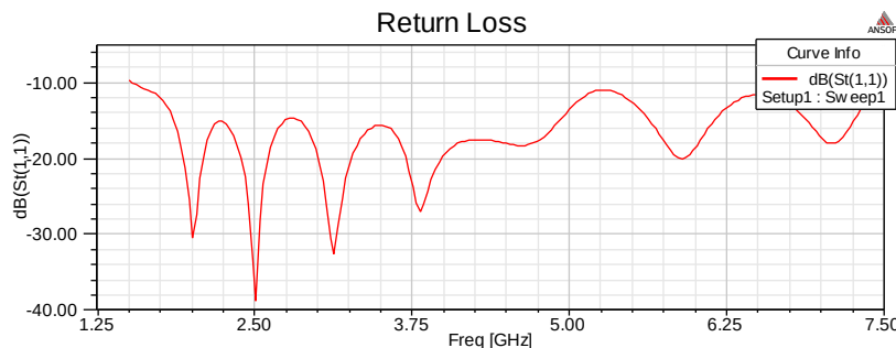
Рисунок 2 – Частотна залежність коефіцієнту відбивання LPDA-антени (коефіцієнту матриці розсіювання S11)
